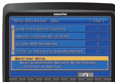
Eco-bedieningsoverzicht
